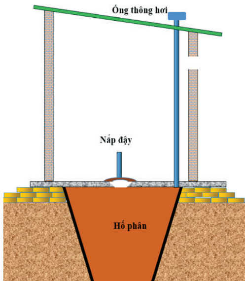
Hình 8. Nhà tiêu chìm có ống thông hơi
